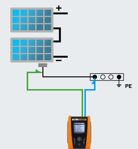
FUNZIONE RPE Schema di collegamento
